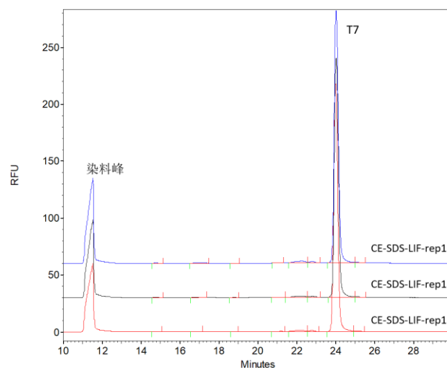
图2. mRNA T7 RNA聚合酶重复性结果（n=3）
