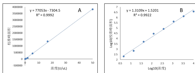
图3. T7 RNA聚合酶的线性图谱。图A为浓度和校准峰面积的线性关系，图B是对横纵坐标取对数log10的结果
