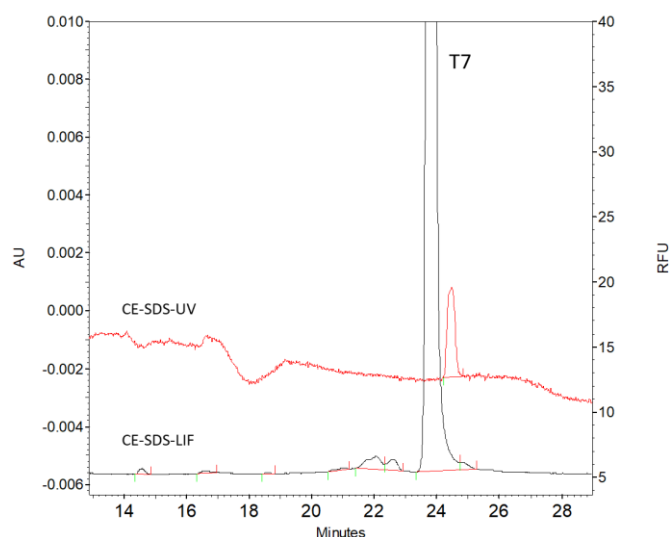
图1. T7 RNA聚合酶纯度电泳图。红色电泳图是CE-SDS-UV结果，响应值对应左侧Y轴；黑色电泳图是CE-SDS-LIF结果，响应对应右侧Y轴。
